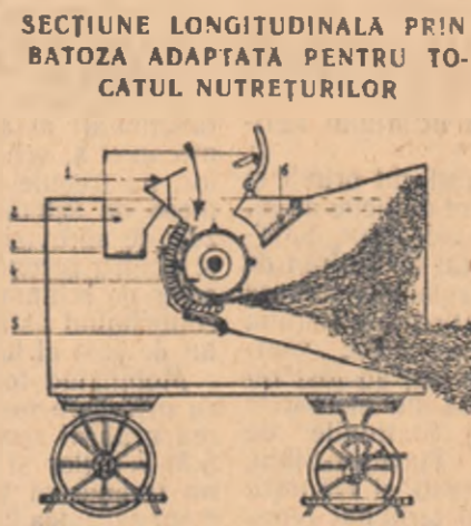
1. Masa cogarului — 2. Locul coșarului — 3. Contrabătător — 4. Tobă — 5. Planul mic inclinat — 6. Scîndura din laja tobei.
