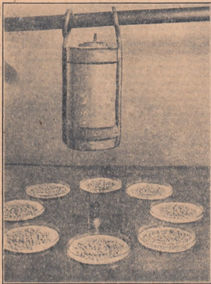
La Institutul de biologie al Academiei de Științe din U.R.S.S. se desfășoară lucrările cercetării pentru folosirea energiei atomice în agricultură. În clădire: O instalație pentru tratarea semințelor cu cobalt radioactiv.
