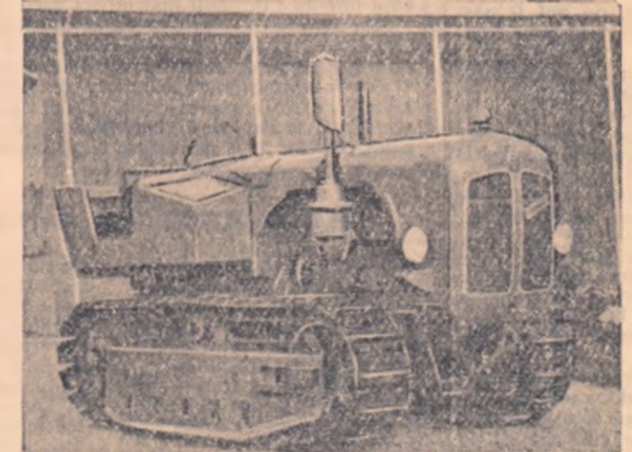
Puternicul tractor pe șenile de tipul „URTRAK”, o frumoasă realizare a industriei de mașini agricole din Republica Democrată Germană. El este înzestrat cu un motor de 62 C. P. și poate fi folosit la cele mai diferite muncile agricole ca: destelînt, detrișari, desfundări în vii, etc.
