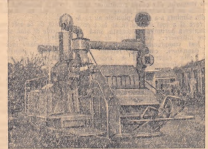
Combina tractată tip „KOMBINUS” pentru recoltat cerealele, produs al fabricii Fortschritt. Această combina poate recolta pe oră o suprafață de 0,75-1 ha. Cerealele recoltate sînt sortate pe două calități, pleava este adunată separat, iar palele sînt lăsate pe cîmp sub formă de baloturi.
