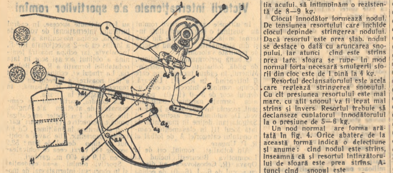
FIG. 1. APARATUL DE LEGARE 1—placă suport innodător, 2—innodătorul propriu zis, 3—brațul aruncătorului de snopi, 4—opritorul de snopi, 5—masa legătorului, 6—brațul declanșatorului, 7—scul, 8—compresorul, 9—întinzătorul de soară, 10—soară, 11—cutia pentru gheme, a 1 —a 2 —ghidajul storii, b—ciocul innodător, c—prînzătorul de soară.
