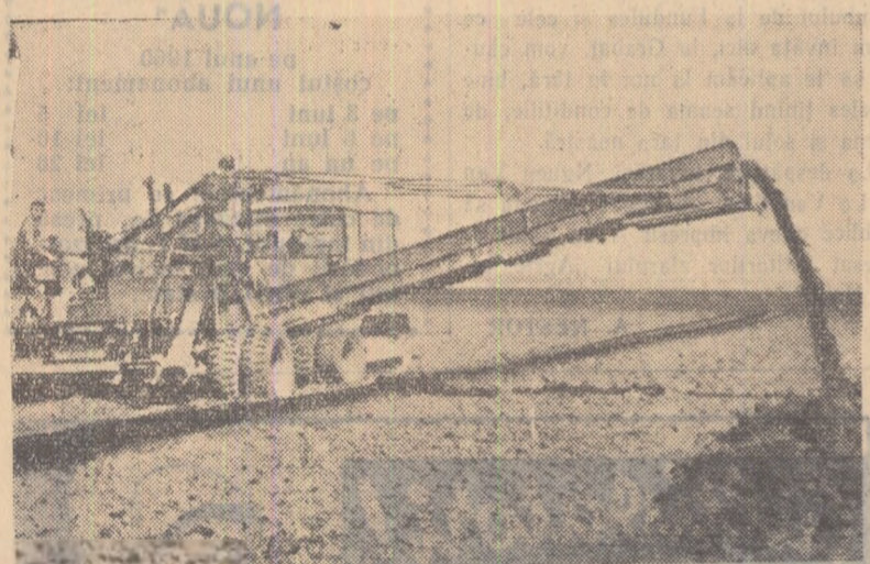
Pe șantierul Stoieniști-Caracal lucrează această mașină sovietică. Ea sapă 1.000 de mc. în opt ore. Adică tot atât cât ar sapa 350 de oameni lucrând manual.
