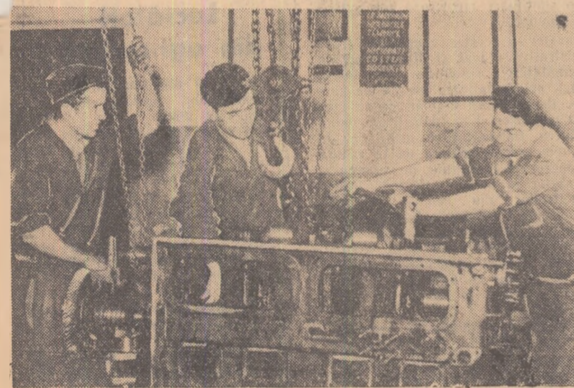
La Centrul mecanic Buzău, repararea motoarelor de tractor se desfășoară cu intensitate sporită. În fotografie: maestrul Tânase Alexandru, împreună cu mecanicii Gună Vanghelie și Gh. Mihai, lucrând la montajul unui motor de tractor greu. (Foto: C. DUMITRU)
