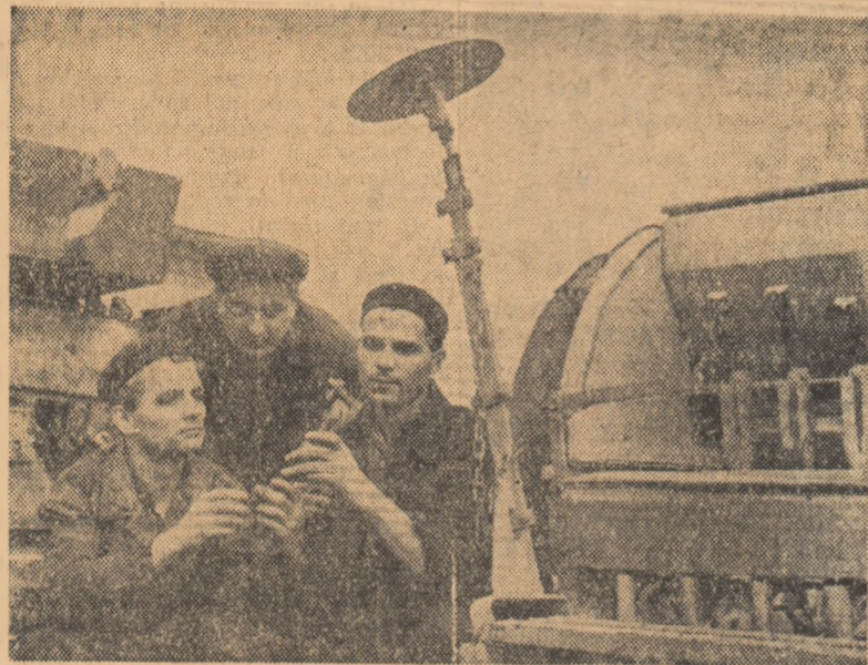
La uzinele „Vasile Roaști” din București, Matrîșterii Victor Băleanu și Marin Grecu din secția a 3-a mașini agricole, consultîndu-se cu șeful brigăzii nr. 1, tov. Achirlian Nicolae, în legătură cu modificarea tijei marcatorei de la semănătoare universale.
