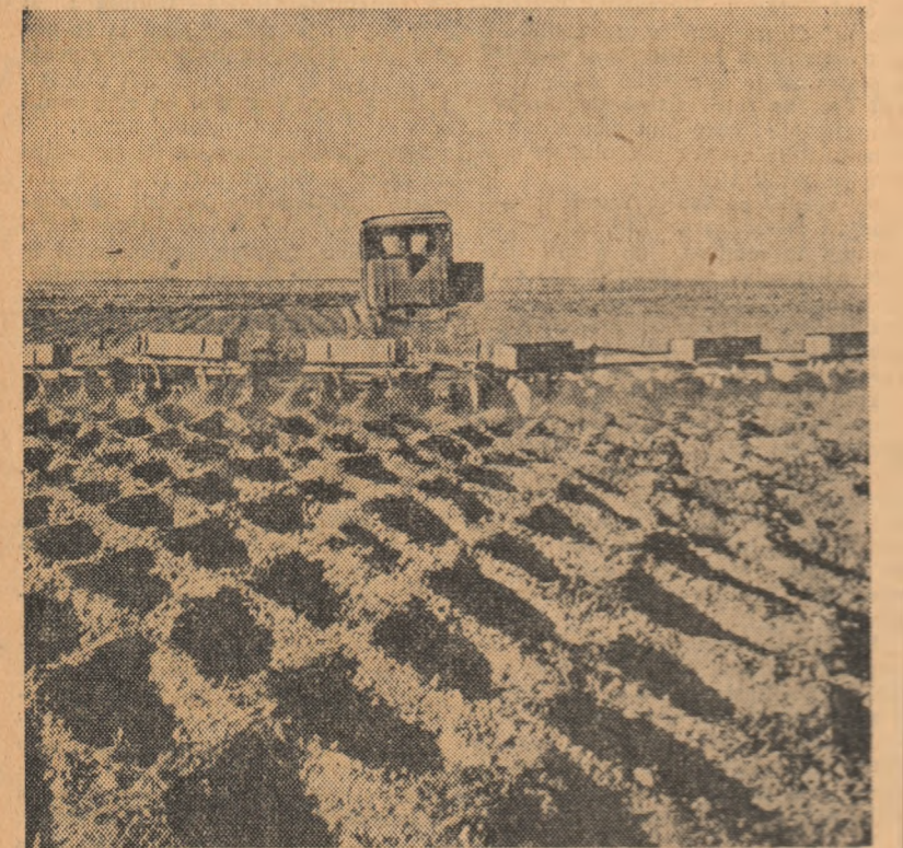
Dezmiriștitor prevăzută cu dispozitiv de săpat cuiburi folosit de Institutul unional de cercetări pentru mecanizarea agriculturii. Mașina face 13.000 cuiburi pe hă care împiedică scurgerea apelor provenite din topirea zăpezii și păstrează umezeala în sol.
