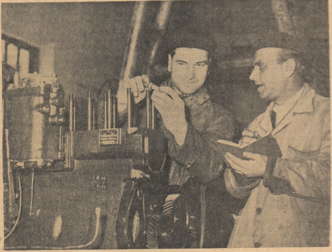
Șeful de atelier Nicolae Cocosilă, împreună cu mecanicul controlor Răduț Vasile, efectuează măsurători la cămășile de cilindru la un motor de tractor.
