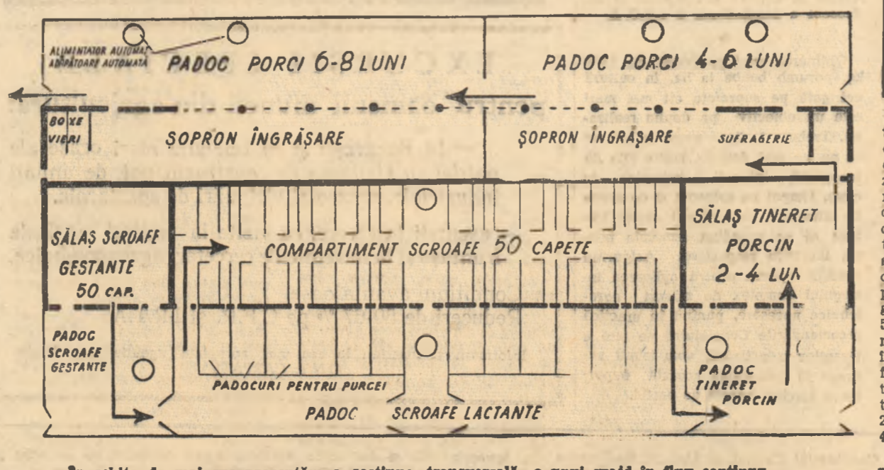
În schița de mai sus prezentăm o secțiune transversală a unui grajd în flux continuu
