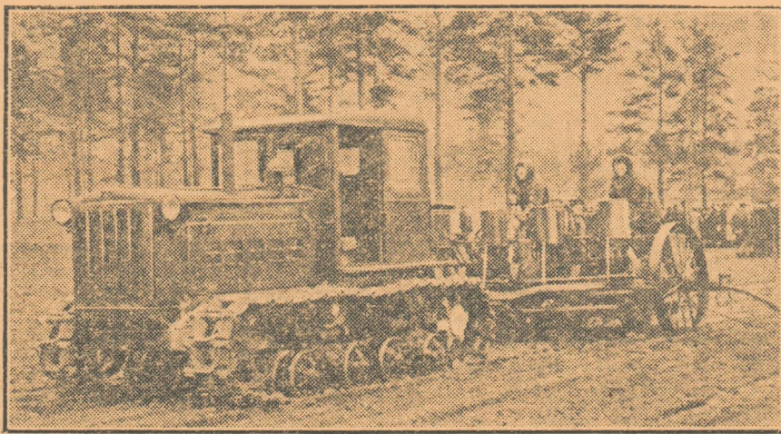
Mașina „S K G-4” pentru plantarea cartofilor în cuiburi pătrate. În acelaș timp ea introduce în cuiburi îngrășăminte minerale.
