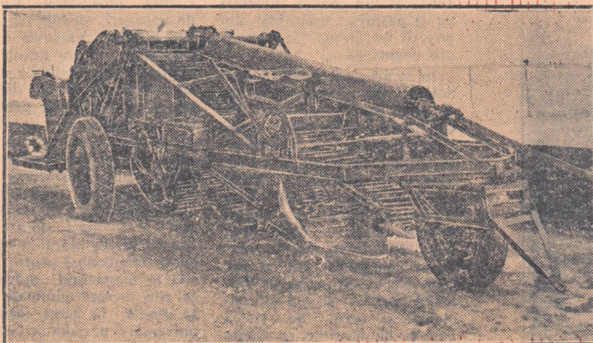
Combina KOK-2 este o nouă mașină pentru recoltarea cartofului. Această combină este pusă în funcțiune de către tractorul DT-54 și este deservită de un tractorist, un mecanic și trei muncitori.
