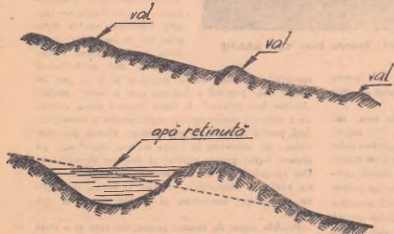
Fig. 1. — Valurile de pămînt sînt lucrări pe care plugarul le poate executa în regiunile de deal, pentru combaterea eroziunii solului. Lucrările constă din mici spinări de pămînt înalte de 30—45 cm. marginile de un șanț în partea de la deal și așezate de-a curmezișul coastei. Ele au rolul de a reține apa de scurgere, forjînd-o să se infiltreze în sol, de unde o iau plantele agricole.
