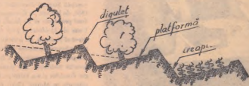
Fig. 3. — Terasele se execută pe coastele foarte mari, unde nu se pot executa mici valuri, nici canale de coastă. Terenul se amenajează în trepte, pe care se plantează pomi sau viță de vie. Înălțimea treptelor terazei poate merge pînă la maximum 4,50 m.
