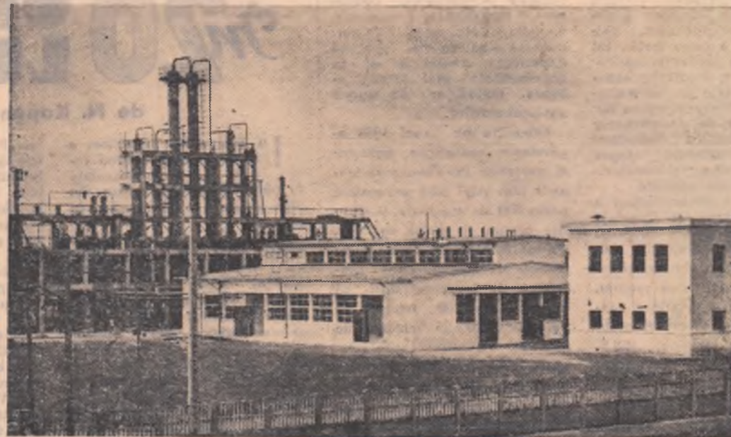
La Brazi, lîngă Ploiești, a intrat în funcțiune o parte a complexului de chimizare a gazelor petrolifere — instalația de fabricare a alcoolilor butilici. Proiectul instalațiilor acestui complex a fost realizat de către IPROCHIM-București, iar aparatura de măsură și control a fost primită din U.R.S.S. și R.D. Germană.
