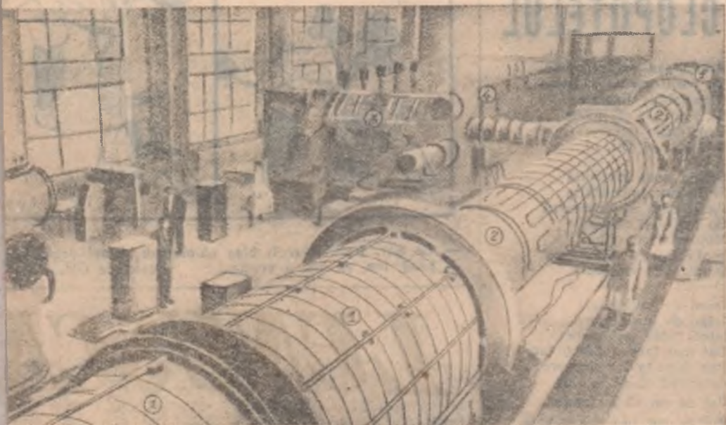
Instalația „Ogra” a Institutului de energie atomică al Academiei de Științe a U.R.S.S. Camera „grei” cu solenoidii îndepărtați. 1. Solenoidii; 2. Camera de rod; 3. Injectorul; 4. Alimentarea cu apă caldă a sursei injectorului.
