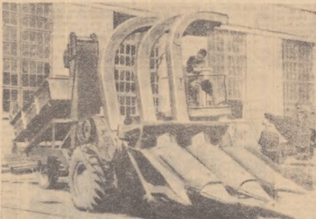
Noua combină de recoltat porumb „KKOH-3” construită de colectivul uzinei „G. I. Petrovski” din Herson. Ea execută tăierea porumbului, desprinderea știuleților, despănșarea, măruntirea tulpinei pentru siloz și încărcarea separată a știuleților și a tulpinei.
