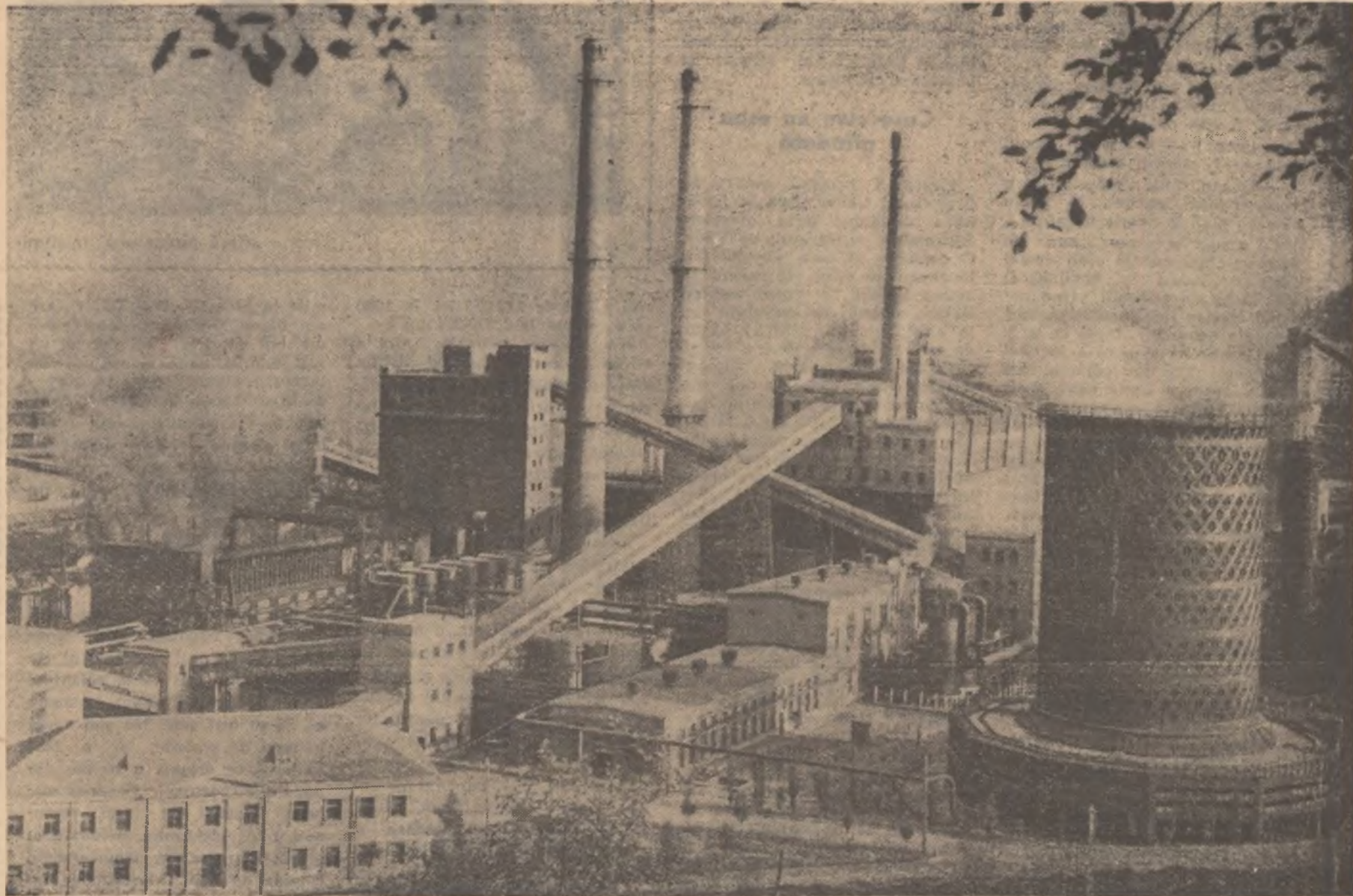
Uzina cocschimică din cadrul Combinatului Siderurgic Hunedoara
