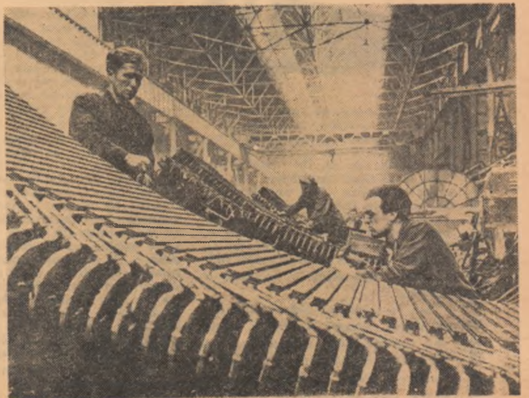
Uzina „Elektrosila” Leningrad: se bobinează un mare stator al unui hidrogenerator pentru o nouă hidrocentrală.
