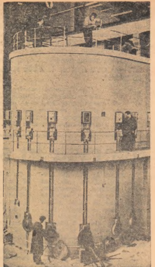
Reactorul atomic de la Salaspils, este primul reactor din Republicile Baltice Sovietice. În clișeu: sala reactorului.
