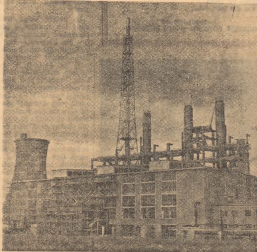
Fabrica de îngrășăminte azotoase Roznov.
