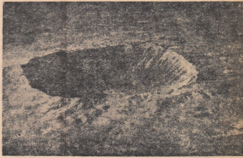
Fig. 4. — Craterul din regiunea Arizona (S.U.A.) format în urma căderii unui mare meteorit.
