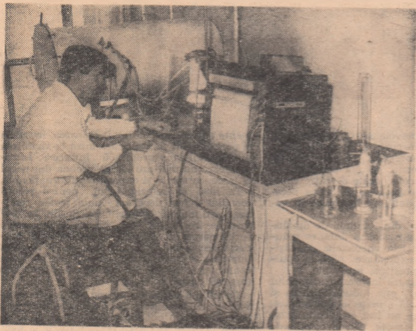
Institutul de Mecanică aplicată din capitală. În laboratorul de metode radioactive, inginerul Ivan Iliuc, cercetător științific, lucrează la etalonarea instalației pentru studii de trecere și uzură cu izotopi în diferite gaze sau în vid
