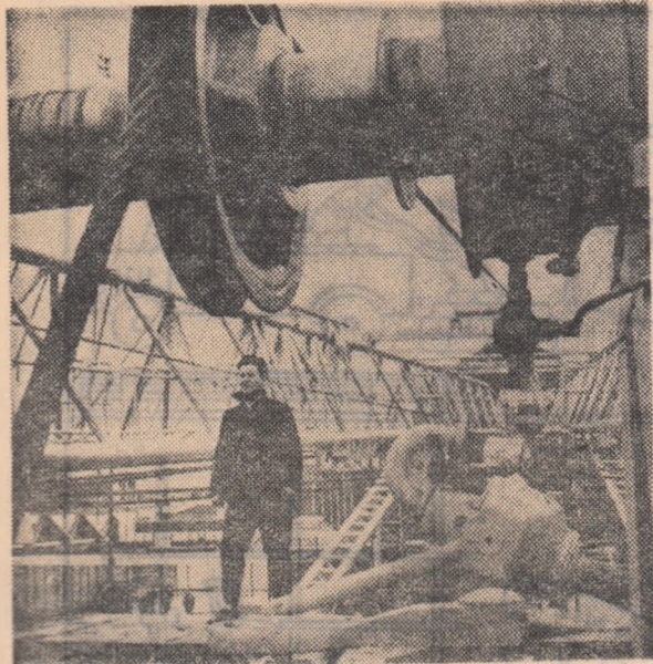
Instalația de foraj românească, în greutate de 360 tone și înaltă de 152 metri, funcționând în întregime automat, s-a bucurat de un deosebit succes la Tîrgul Internațional de la Leipzig
