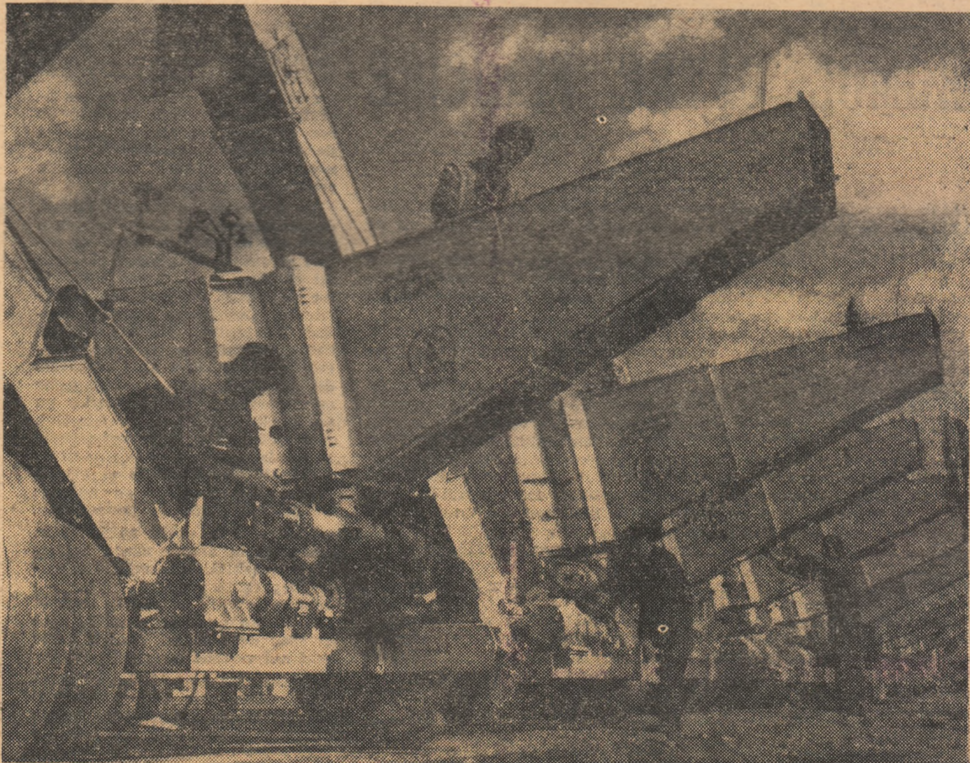
La Uzina „Semănătoarea” din Capitală, se face o ultimă verificare a unui lot de combine C.T. 2 R. înainte de a fi expediate
