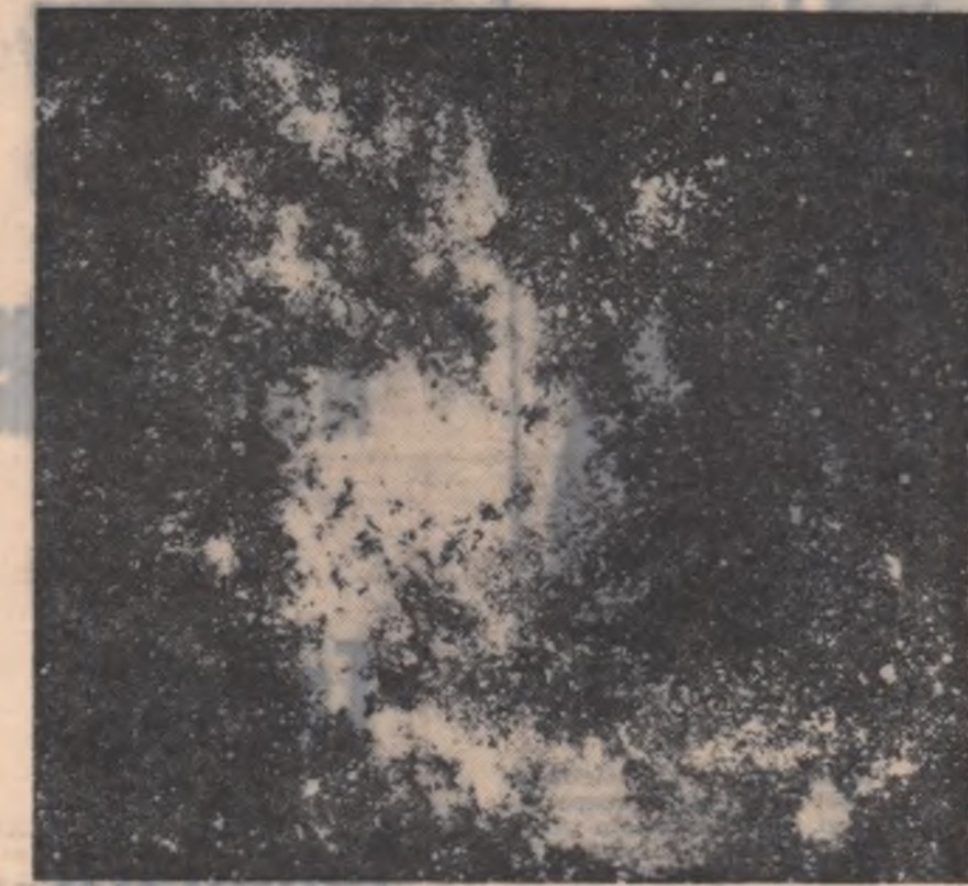
Una din miliardele de lumi existente în Univers: Galaxia spirală din constelația Triunghiului aflată la o depărtare de Pământ de aproximativ 2 milioane de ani-lumină.
