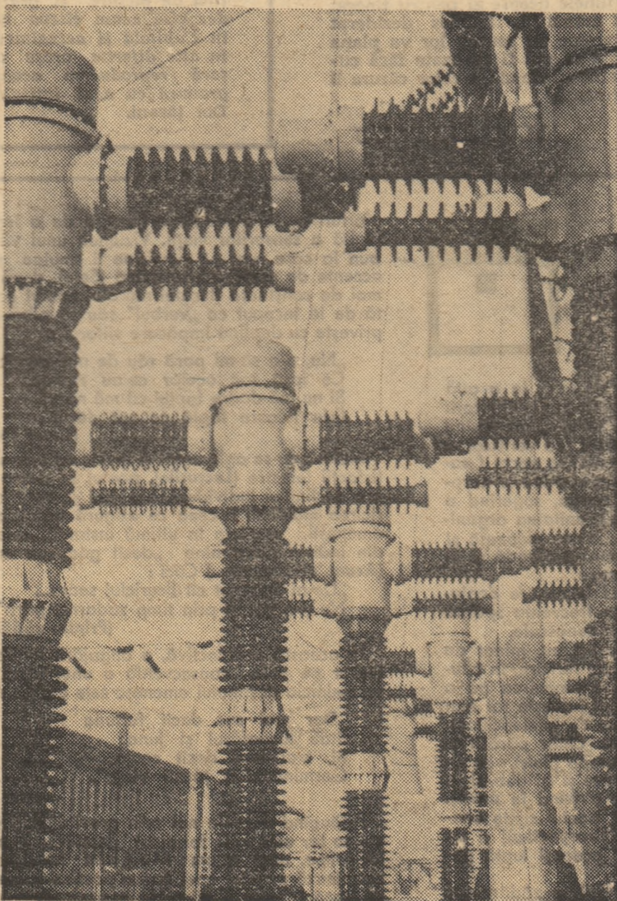
Transformatori de înaltă tensiune
