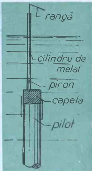
Fig. 2 Baterea pironelor sub apă
