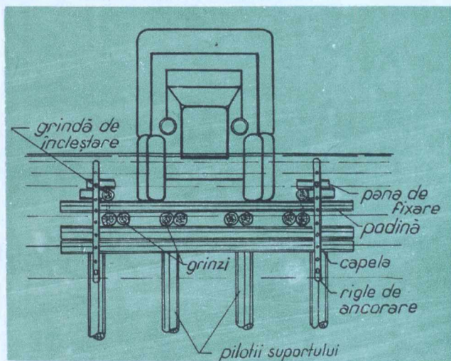
Fig. 4 Secțiune transversală în dreptul unui suport
