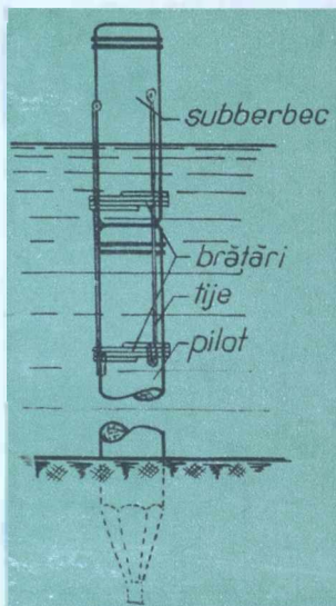
Fig. 1 Baterea piloților sub apă
