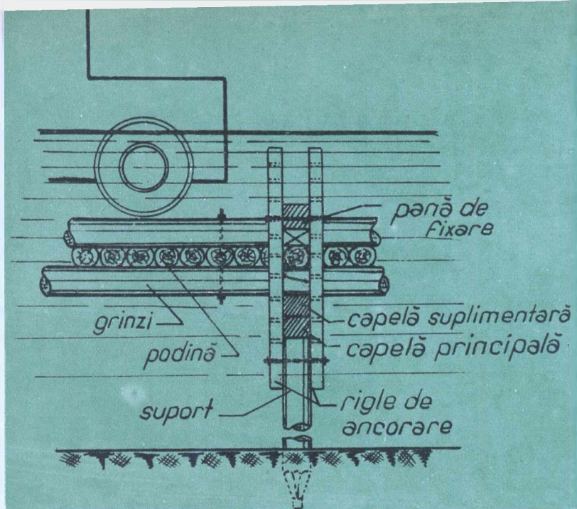
Fig. 3 Prinderea suprastructurii de suport
