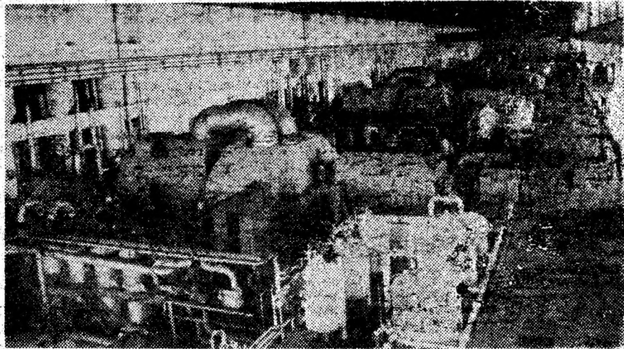
Sala mașinilor
