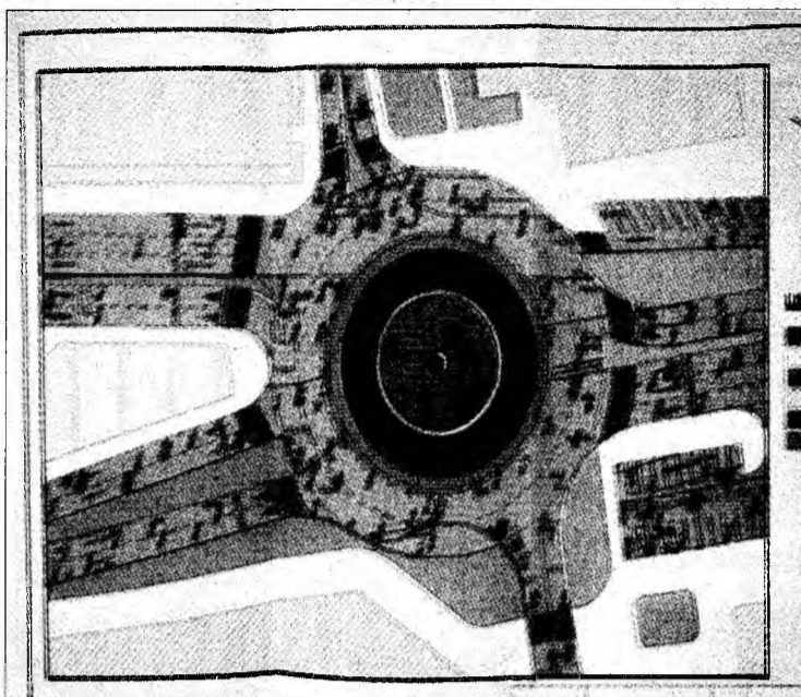
Proiect al sensului giratoriu de la Lido
