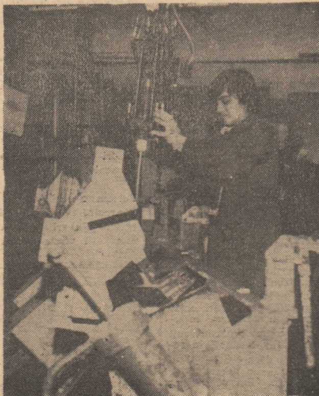
I. C. Orăștie — secția poliuretani. Tînăra operatoare Angela Cățineanu lucrează la o mașină de confecționat bord pentru autoturismul ARO-10.
