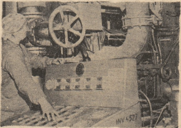
I.M.C. Bircea, atelierul polistiren. Vedere de la tabloul de comandă al mașinii de format blocuri polistiren.
