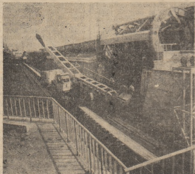
Activitate susținută, neîntreruptă, în gospodăria de cărbune a C.T.E. Mintia. În prim-plan: mașina cu roată cu cupe de preluat cărbune din depozit și instalația de culbure a vagoanelor.
