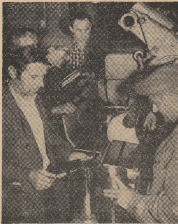
I.A.C.R.S. Hunedoara. Maștrii Constantin Diaconescu și Nicolae Deliu au gândit și pus în lucru un procedeu tehnic care permite recuperarea și reutilizarea cămășilor cilindrică de la motoarele autocamionelor „TATEA”. Acest lucru contribuie la economii de aproximativ 2.000 lei la reparația unui motor. Foto NICOLAE GHEORGHIU
