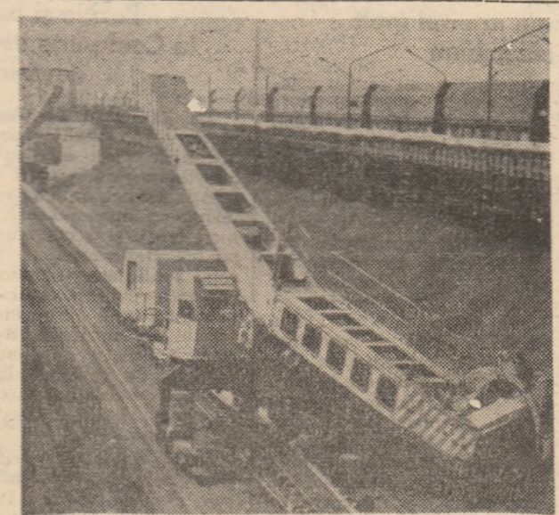
C.T.E. Mintia — gospodăria de cărbune. Mașina cu roată cu cupe LWK 251, de preluat cărbune, alimentează continuu benzile transportoare, care duc hrană indispensabilă la cazane.
