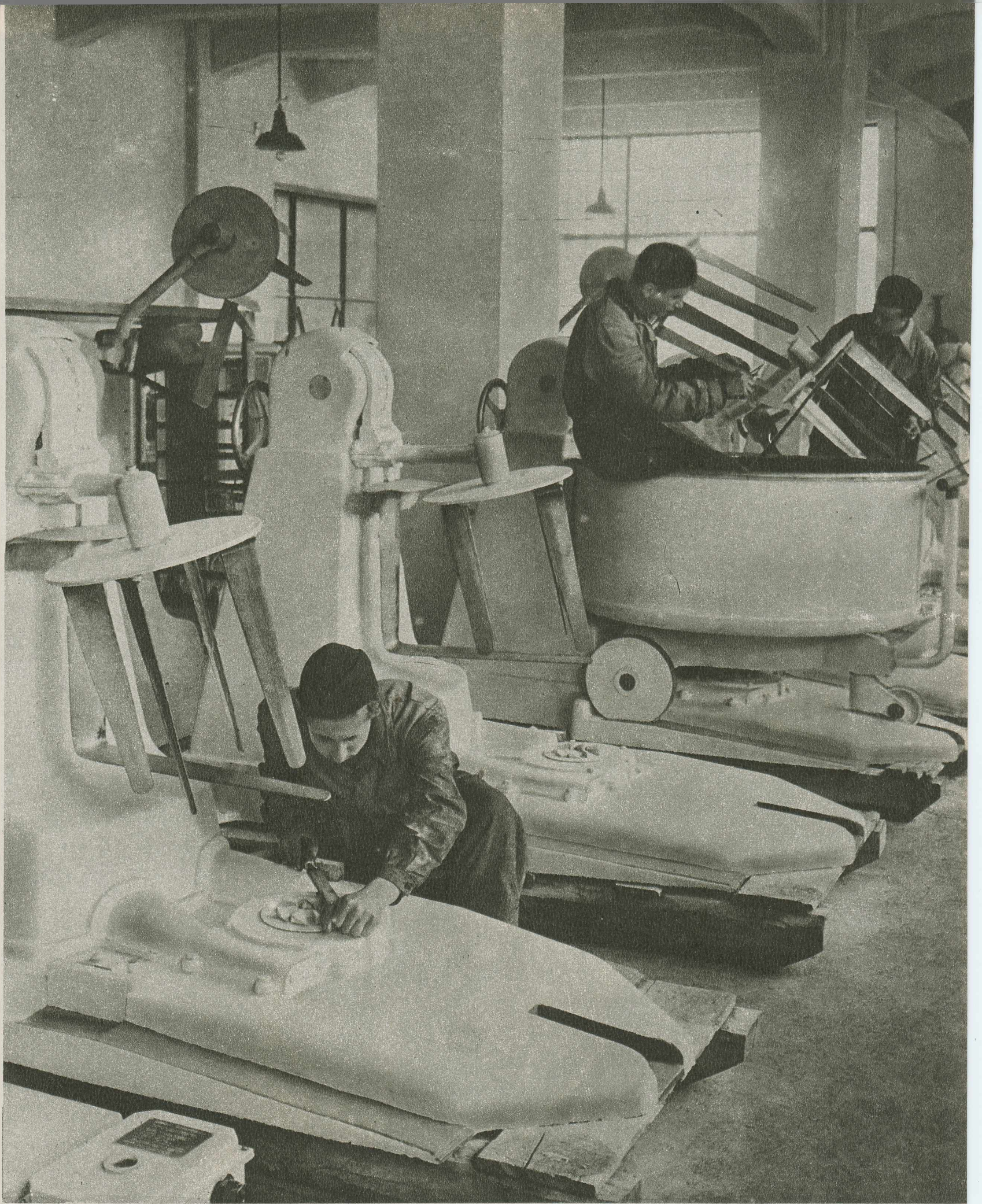
Fabrica „Tehnofrig” din Cluj produce utilaj modern pentru întreprinderile industriei noastre alimentare. În fotografie: se assemblează malaxoarele de frământat coca pentru plăci.
