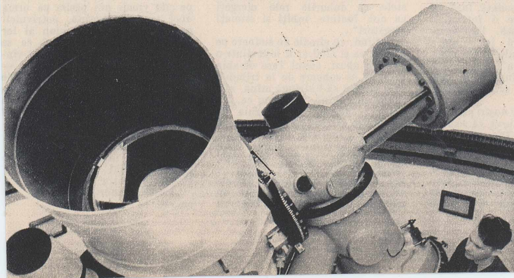
Telescop cu menisc de 50 cm. construit după sistemul savantului sovietic D. D. Maksutov
