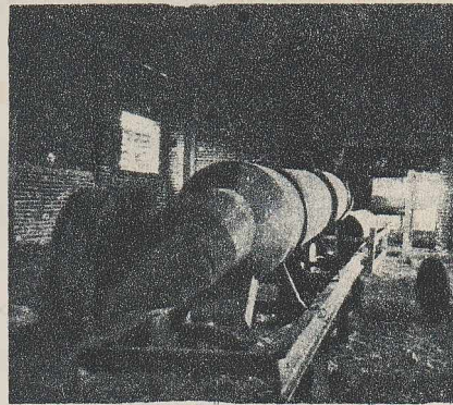
Mașina de granulat îngrășăminte.
