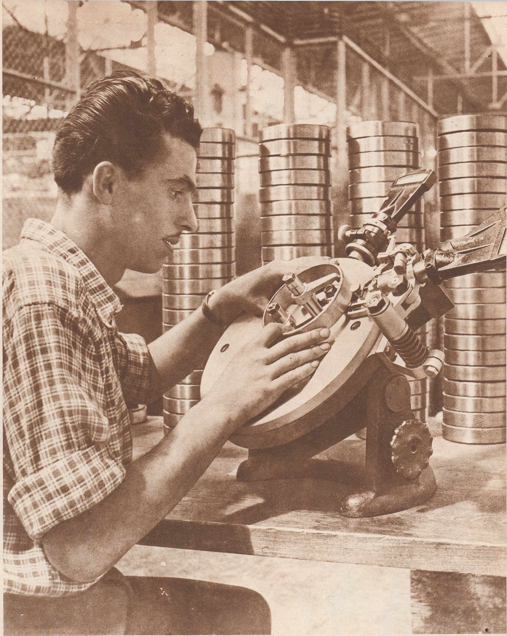
Aspect de muncă de la fabrica de rulmenți din Moldova, construită în anii regimului democrat-popular: muncitorul utemist Ilie Predelcu, lucrând la aparatul pentru controlul căilor de rulare de la rulmenții conici. Sînt din ce în ce mai mulți muncitorii care, răspunzînd chemării Partidului, își ridică neîncetat nivelul tehnic și științific.
