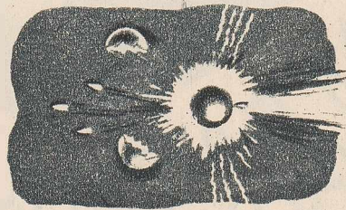
Dezagregarea nucleului de uraniu sub acțiunea neutronului. Nucleul se sfarmă în două părți. Cu acest prilej apar doi-trei neutroni noi.
