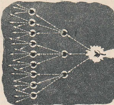
Un neutron provoacă o reacție în lanț, care cuprinde un număr enorm de atomi.
