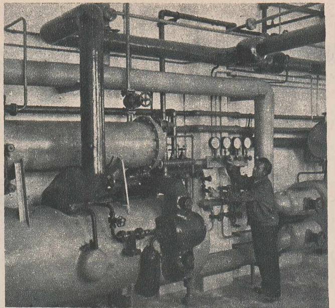
⬆ Patria noastră a primit încă un dar prețios: la Remetea a intrat în funcție prima fabrică de lapte-praf din țară. În fotografie: Ștefan Axinescu, șef de schimb la stația de reglare, controlează amestecul lichid din condensator.
