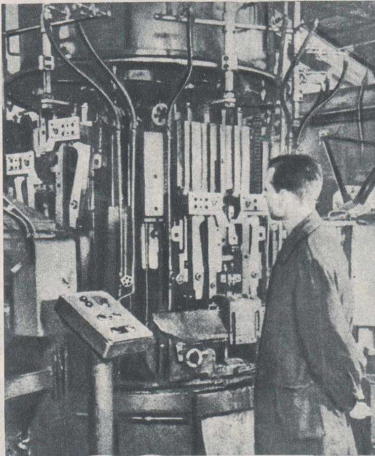
Lucrătorul-controlor supraveghează modul de funcționare a mașinii automate de turnat.
