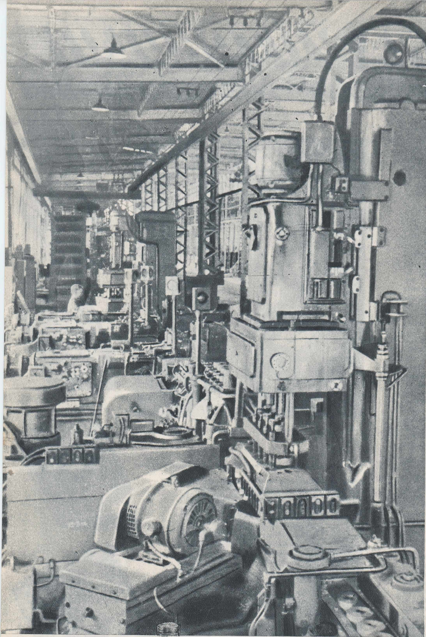
O minune a tehnicii: un singur lucrător dirijează întreaga activitate a liniei automate a uzinei de pistoane pentru automobile.
