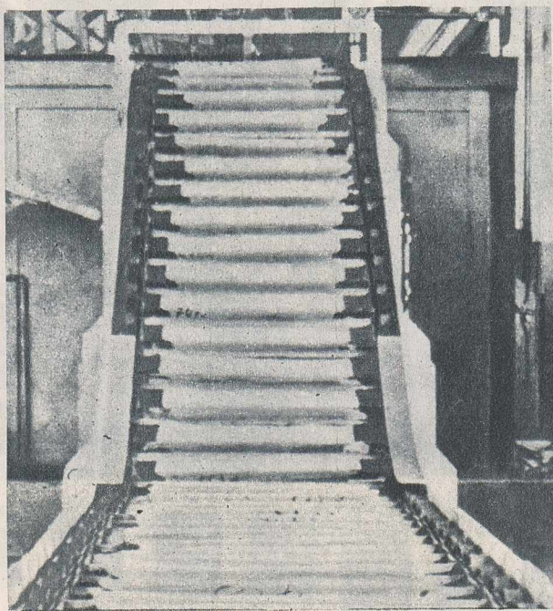
Bandă rulantă care transportă automat bare de aluminiu la gura cuptorului de topire.
