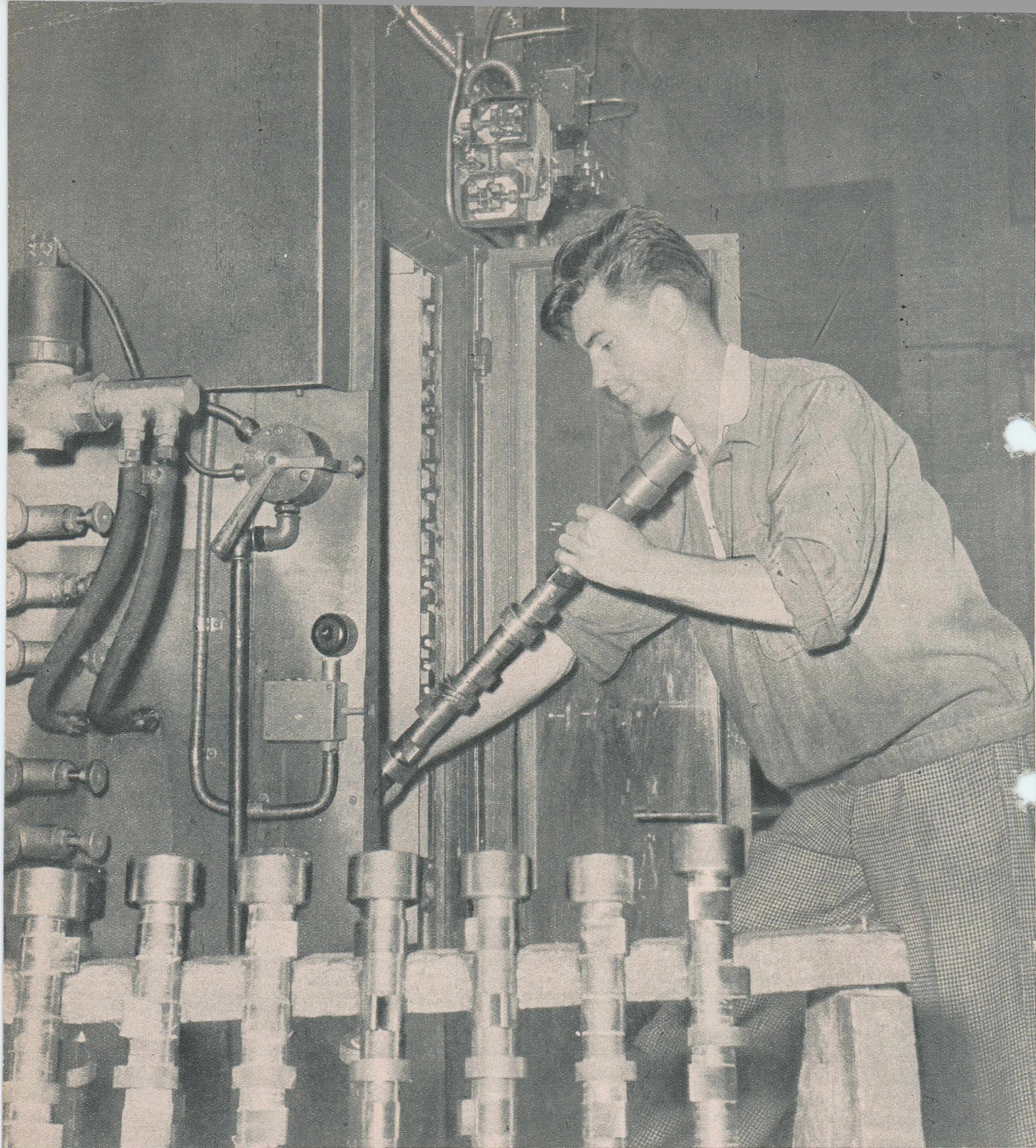
Tînărul muncitor Vasile Duda, de la uzinele „Steagul Roșu” din Orașul Stalin, a deprins repede să minuiască noua mașină de căltre prin curenți de înaltă frecvență a axelor cu came, construită de un colectiv de muncitori, ingineri și tehnicieni din uzină.
