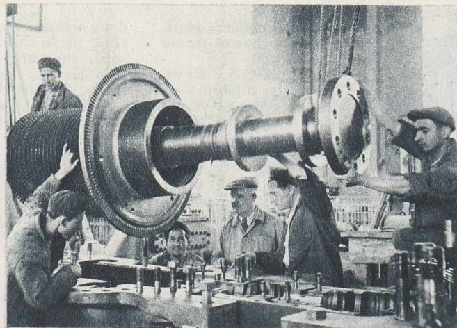
Acest turbo-generator va mări mult capacitatea de producție a fabricii. El a fost lucrat în R.P. Ungară și este montat la noi cu sprijinul specialiștilor maghiari.
