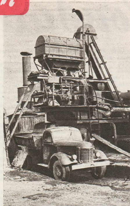
Betonul asfaltic este descărcat în autocamionul basculant, care îl transportă spre șoseaua în reconstrucție...
