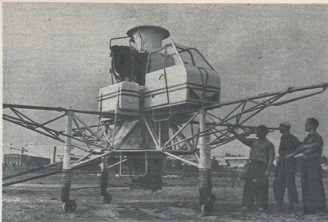
Turboplanul sovietic sau „masa zburătoare”, cum este denumit, constituie un prim pas îndrăzneț, pe calea creării ur aviației care nu are nevoie de aerodroame. Deși aparatul nu are nici aripi, nici elice, el se comportă excelent în aer.
