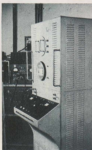
SPECIALIȘTII DE LA INSTITUTUL DE FIZICĂ ATOMICĂ al A.C.R.P.R. au realizat un nou aparat pentru studierea radiațiilor nucleare: Aparatul de amplitudine cu memorie electronică. Construit pentru prima oară în țara noastră și executat în întregime din proiecte originale, acest aparat analizează șase la măsurarea energiei gama ale diferiților izotopi prin reacția atomică. Cu ajutorul noului aparat se deosebește cu mare precizie puritatea elementelor care formează obiectul studiului și care nu poate fi stabilită în alte moduri.
