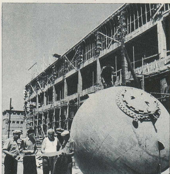
UNUL DIN FIERBĂTOARELE SFERICE cu care va fi utilat combinatul de celuloză și cartoane din stuf de la Chișcani-Brăila face obiectul de studiu al montorilor. El primește lămuriri de la maestrul coordonator Enache Petre asupra felului cum va trebui montat.
