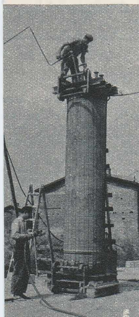
FURURILE DE PRESIUNE confectionate din beton pre- comprimat sunt mai avan- țate, nefiind supuse coro- ziunii. Institutul de cercetări pen- tru construcții, materiale de construcții și lemn cerce- ază posibilitățile de înlocu- irea a unor materiale scumpe altele mai ieftine, având aceiași rezistență.
