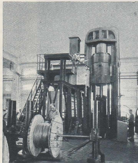
FABRICA „ELECTROCABLUL” din Capitală a fost dotată cu noi agregate și utilaje de mare capacitate. Printre acestea se află și presa de plumb cu ajutorul căreia se montează plumbul la cablurile de forță și telefonice.
