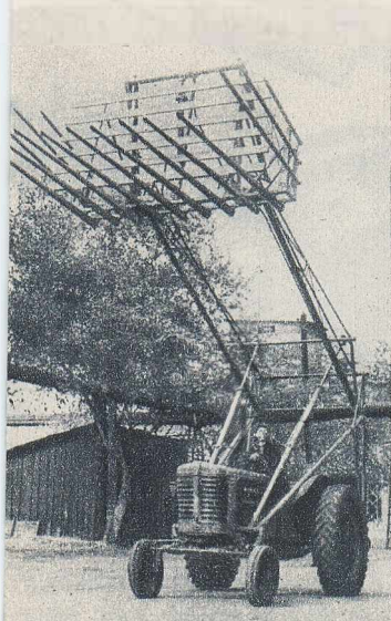
MASINA DE „FABRICAT”... CLĂI DE N. La uzina de construcții de mașini agricole „Uhtomski” din Liubert, ținea Moscova, se produce în serie dispozitiv hidraulic pentru clăi de N. Noua mașină poate ridica o câpșă greutate de 500 kg și o poate depune supra clăii de fin la o înălțime de metri.
