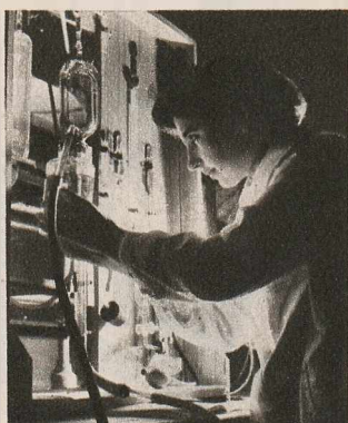
UN ASPECT din laboratoarele uzinelor „23 August” din Capitală: cu ajutorul unui aparat special, se determină procentajul de carbon și de sulf din oțeluri și fontă.
