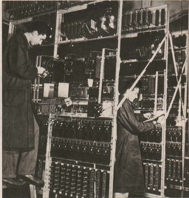
S.C.B. — semnalizare, centralizare, bloc de linii automate — se numesc pe scurt echipamentele pentru automatizarea stațiilor C.F.R. Complicatele aparate sînt produse de colectivul uzinelor „Grigore Preoteasa” din Capitală, care și-a propus ca în anul 1959 să producă noi tipuri de asemenea echipamente. Iată-l pe nunciitorii Olimp Melinte și Paul Mihăilescu, lucrînd la asamblarea ramelor de alimentare pentru S.C.B.
