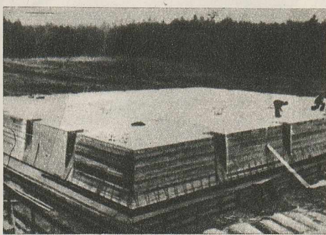
La Rheinsberg, în nordul Berlinului, se construiește prima centrală atomoelectrică a R.D. Germane, care va folosi uraniu greu 235 și va avea o putere de 70 megawați — ce va putea fi dublată. În timp ce în R.F.G. se înzestrează Bundeswehrlu cu arma atomică, R.D. Germană, prin construirea acestui important obiectiv, dă o nouă dovadă a dorinței poporului german de folosire a energiei atomice în scopuri pașnice.
