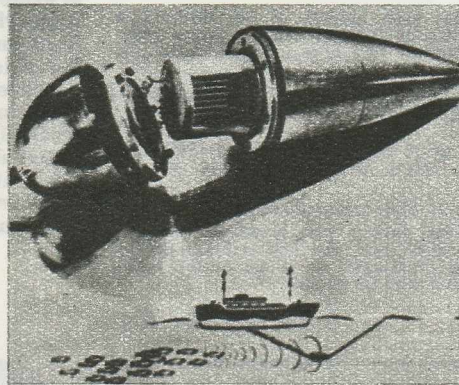
"HIDROFON PIEZOELECTRIC" se numește acest aparat ultrasonic realizat la Institutul de acustică al Academiei de științe a U.R.S.S. Aparatul a fost folosit cu succes la depistarea bancurilor masive de pești.
