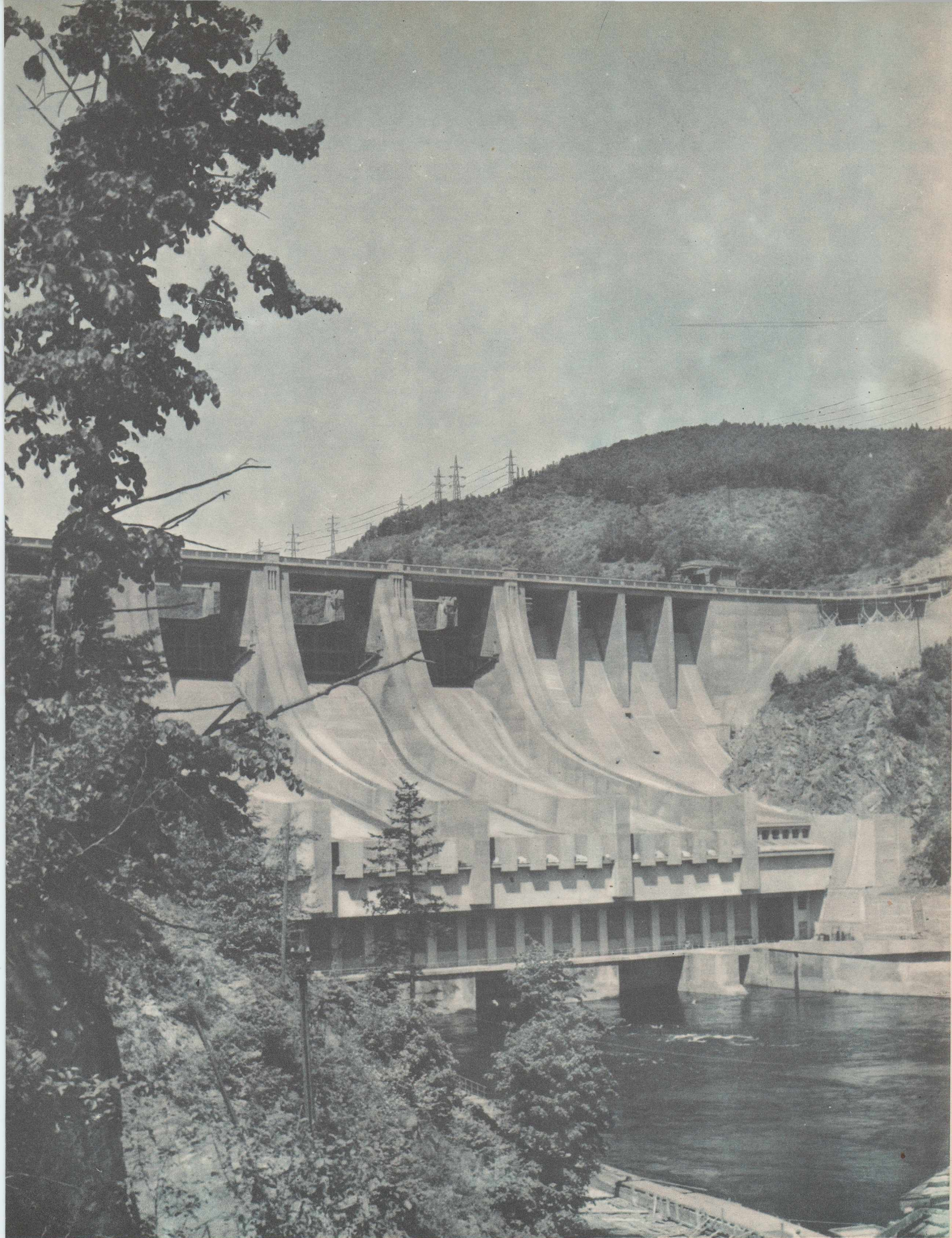
idrocenrala de la Slapy este una din marile construcții ale Cehoslovaciei noi, expresie a înaltului nivel al tehnicii din țara vecină și prietenă. In fotografie: barajul hidrocentralei
