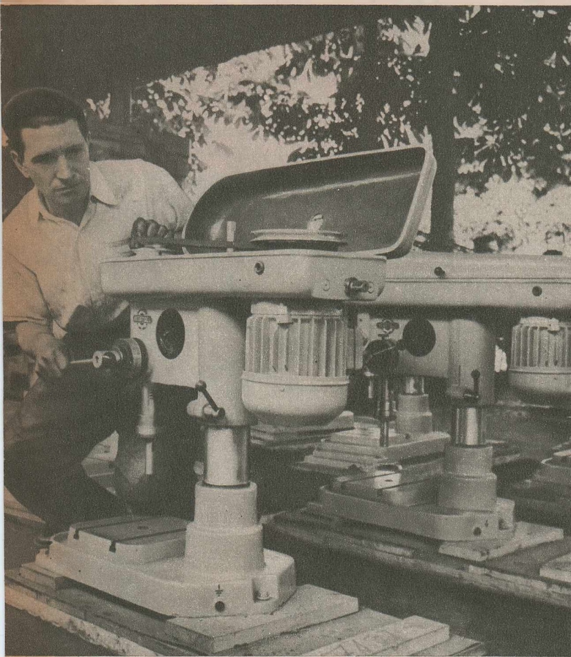
Întreprinderea „Înfrățirea” din Oradea execută o gamă întreagă de mașini-unelte. Modernizarea procesului de producție este principala grijă a întregului colectiv. Prin procedeele de mecanizare în curs de aplicare se vor economisi 150 tone de metal. În fotografie: un nou lot de mașini de găurit „A-3” se află la ultimul control de calitate.
